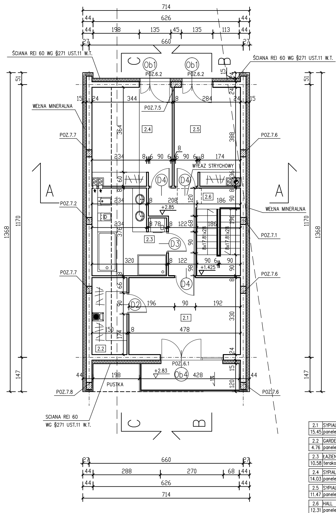
RZUT PODDASZA 1:100
