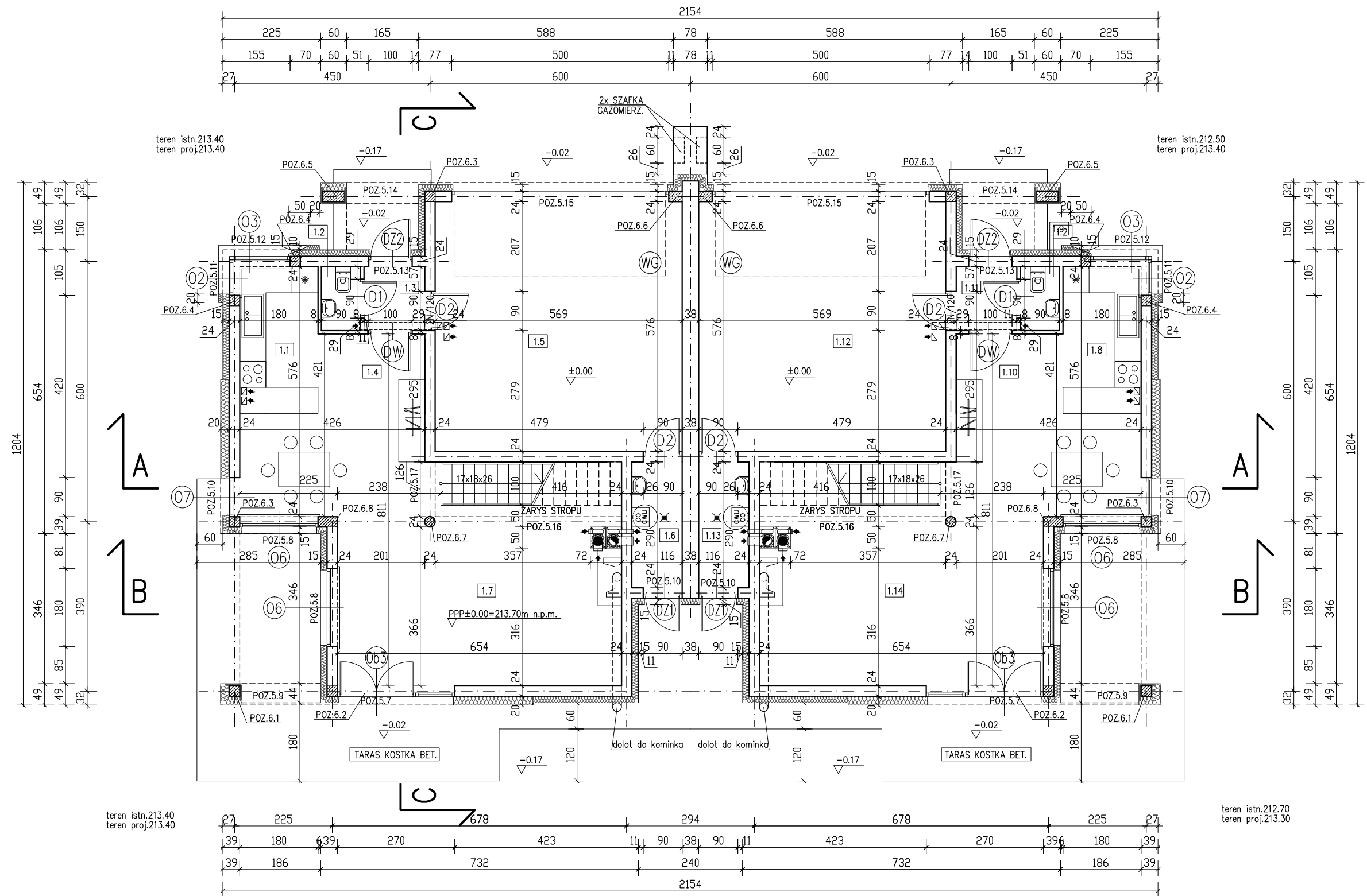
RZUT PARTERU 1:100
