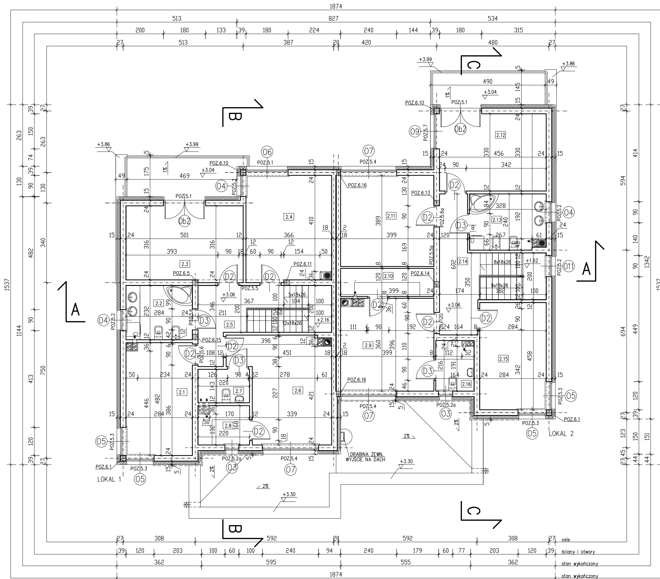
RZUT PIĘTRA 1:100
